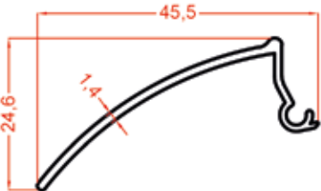
1217 0.240 Kg/m
