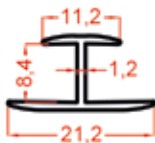
1528 0.115 Kg/m
