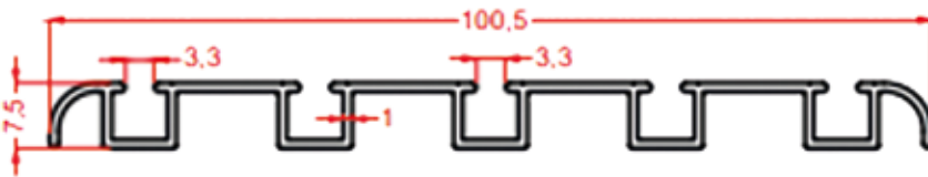
1627 0.510 Kg/m
