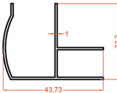
1637 0.341 Kg/m
