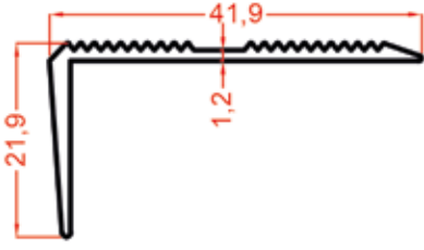
1515 0.261 Kg/m
