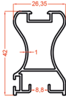
1441 0.458 Kg/m
