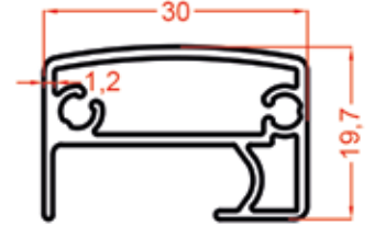
1633 0.400 Kg/m
