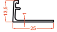
1408 0.125 Kg/m
