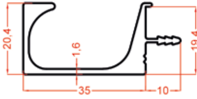
1435 0.566 Kg/m
