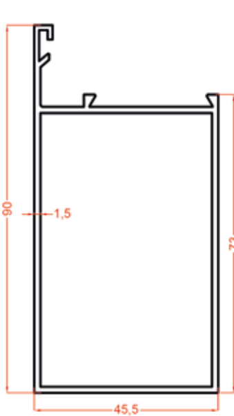
337 0.599 Kg/m
