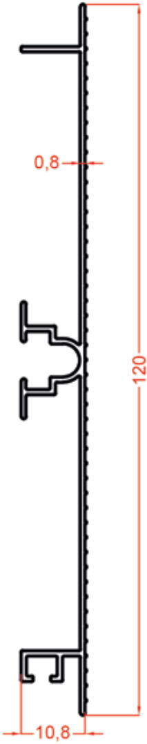
1440 0.436 Kg/m
