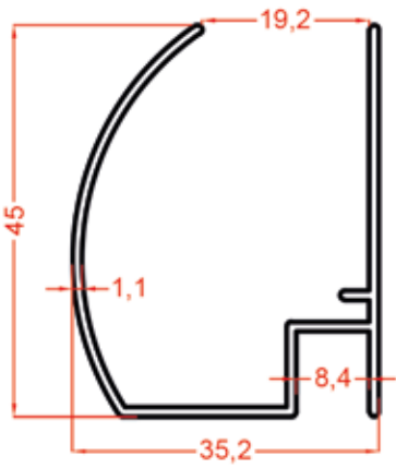
1344 0.405 Kg/m
