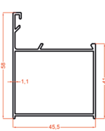
239 0.495 Kg/m
