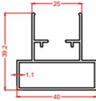
296 0.516 Kg/m
