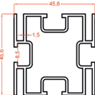
1220 1.160 Kg/m
