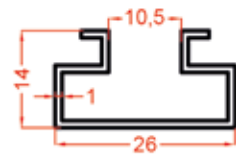
1429 0.194 Kg/m
