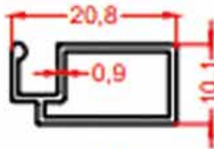
162 0.152 Kg/m
