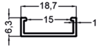
1749 0.85 Kg/m
