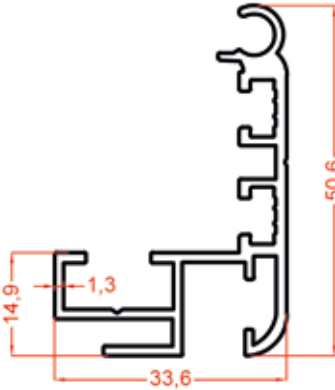
1212 0.644 Kg/m
