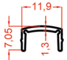
390 0.069 Kg/m
