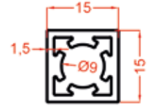
1404 0.321 Kg/m
