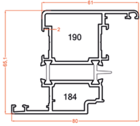
190 0.950 Kg/m 184 0.751 Kg/m
