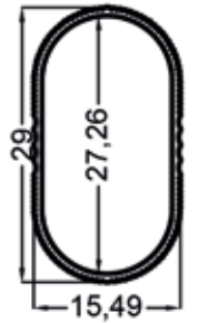
1757 0.156 Kg/m
