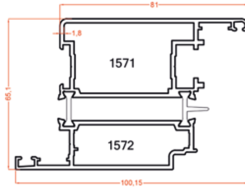
1571 1.179 Kg/m 1572 0.894 Kg/m
