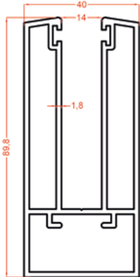
355 2.068 Kg/m
