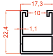
1584 0.245 Kg/m
