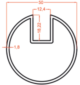
294 0.749 Kg/m
