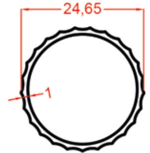
1512 0.217 Kg/m
