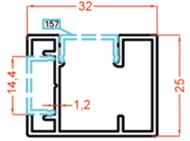
159 0.388 Kg/m
