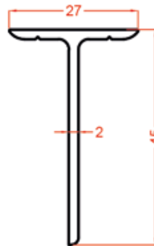
1218 0.374 Kg/m
