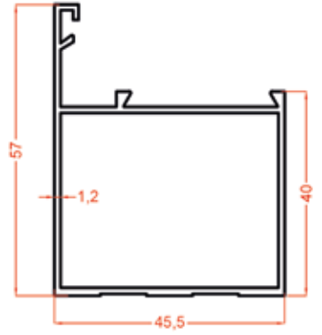
220 0.674 Kg/m
