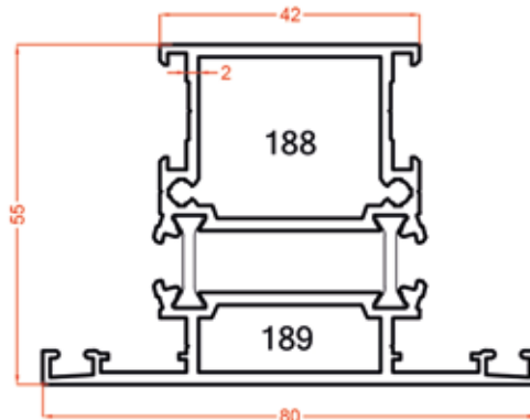
188 0.821 Kg/m 189 0.874 Kg/m
