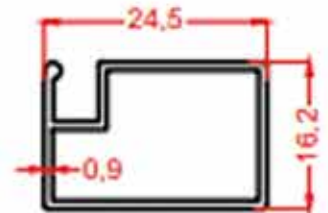
163 0.210 Kg/m
