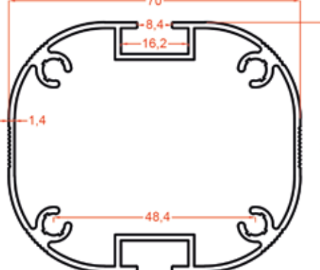
397 1.309 Kg/m
