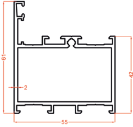
191 1.214 Kg/m
