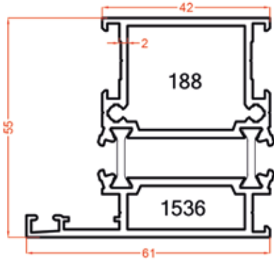
188 0.821 Kg/m 1536 0.745 Kg/m
