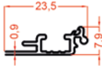
1208 0.122 Kg/m
