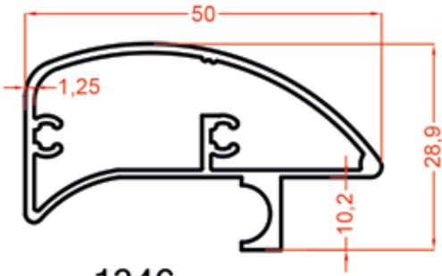
1346 0.569 Kg/m
