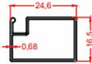
1482 0.161 Kg/m
