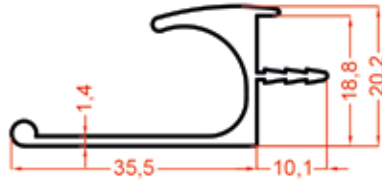
1427 0.430 Kg/m
