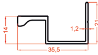
1430 0.287 Kg/m
