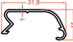
1207 0.114 Kg/m
