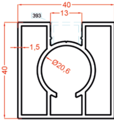
392 1.003 Kg/m
