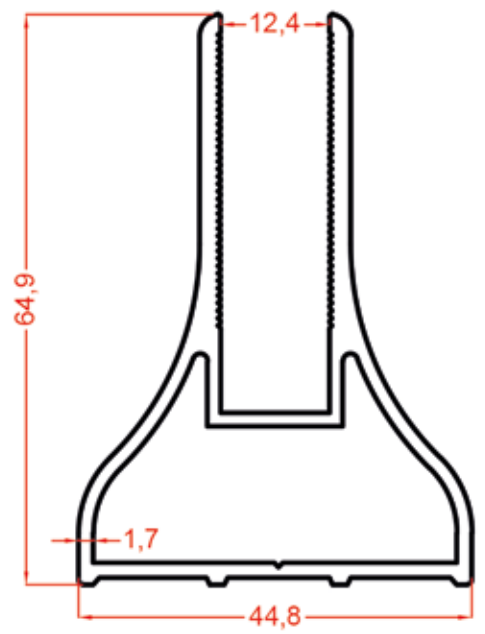
385 1.120 Kg/m
