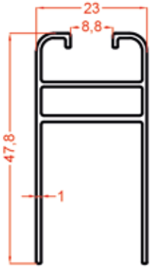
1537 0.430 Kg/m
