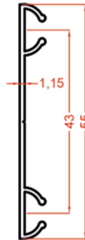
1436 0.239 Kg/m
