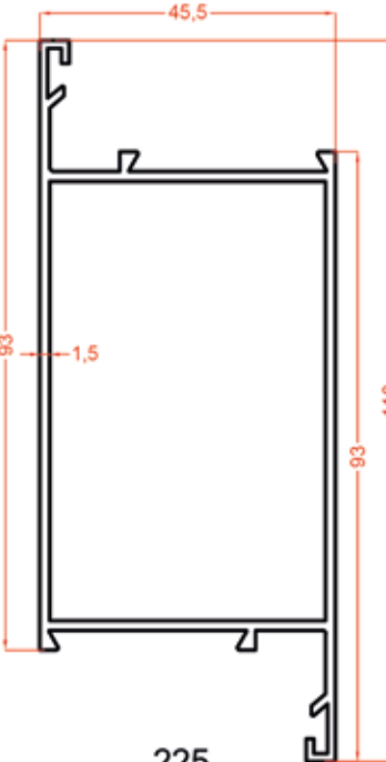
225 1.190 Kg/m
