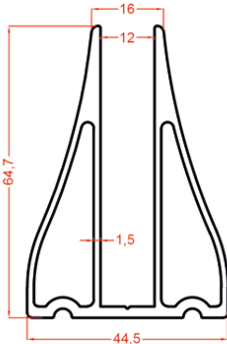
198 1.398 Kg/m
