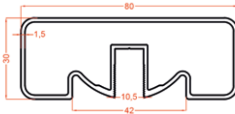
1402 1.084 Kg/m
