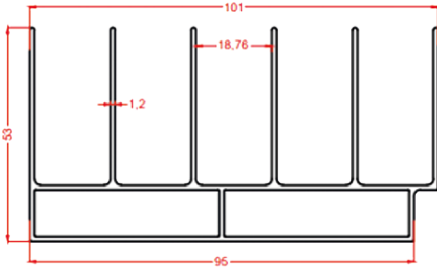
1625 1.525 Kg/m
